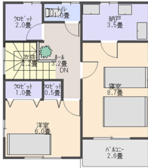
2F間取り
