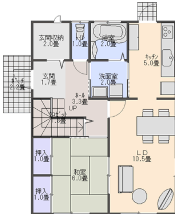
1F間取り
