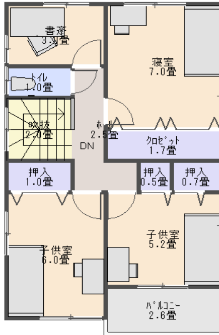
2 F 間取り
