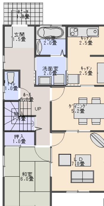
1 F 間取り
