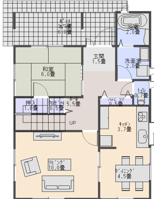
1 F 間取り
