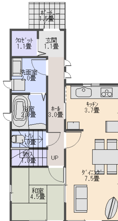
1 F 間取り
